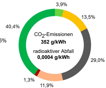
Zum Vergleich: Stromerzeugung in Deutschland im Jahr 2019*
